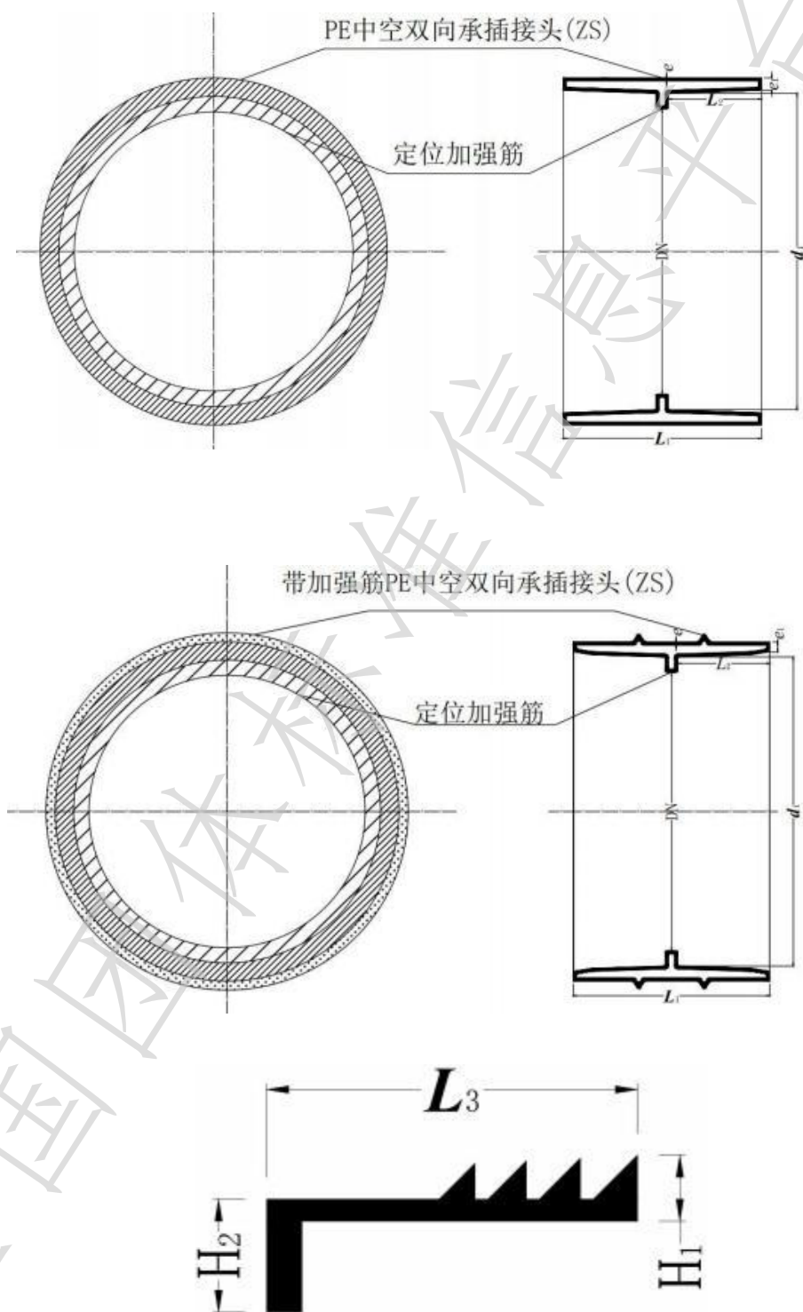
图3 PE中空双向承插接头 (ZS) 及L形多峰橡胶密封圈
