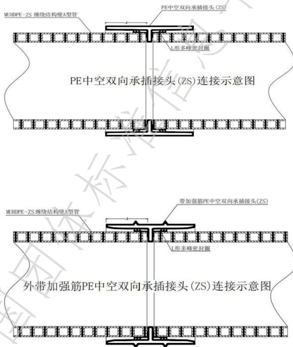
图 2 管材中空双向承插接头（ZS）连接示意图
