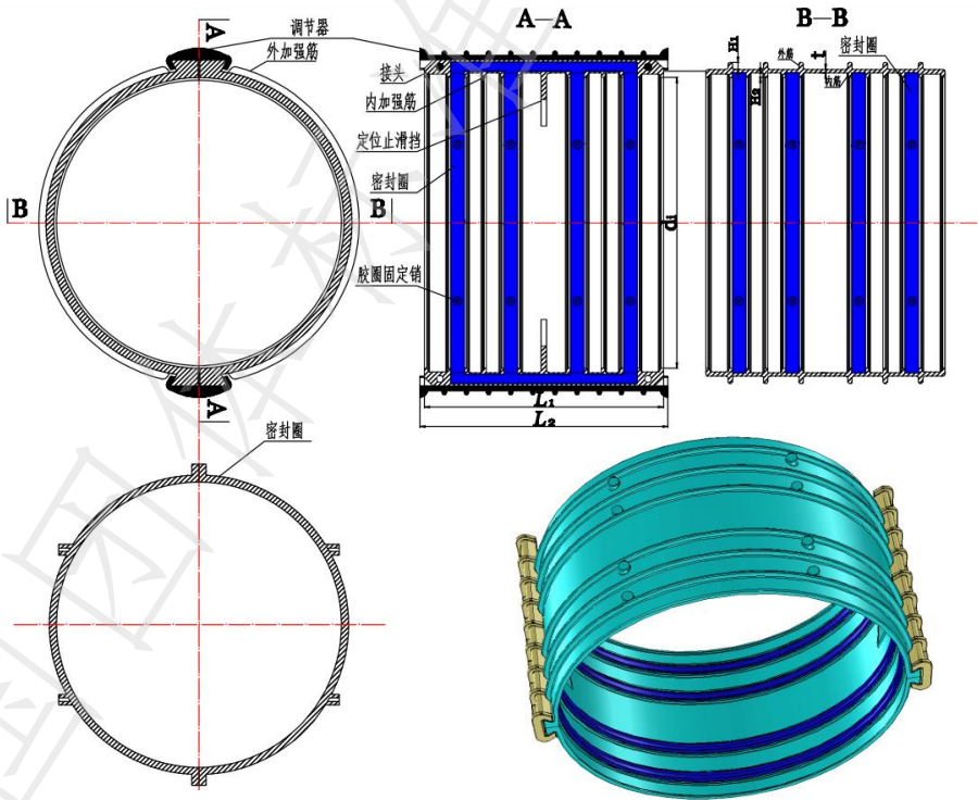
图 2 管材装配式连接示意图
