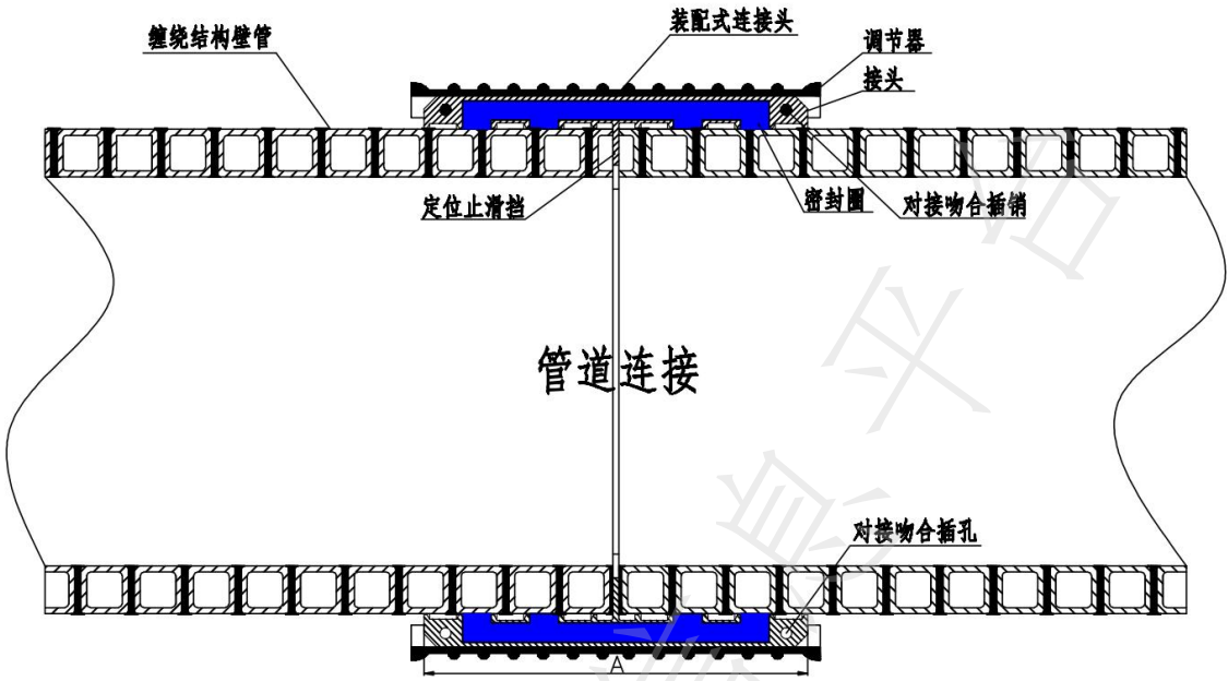
图 2 管材装配式连接示意图
