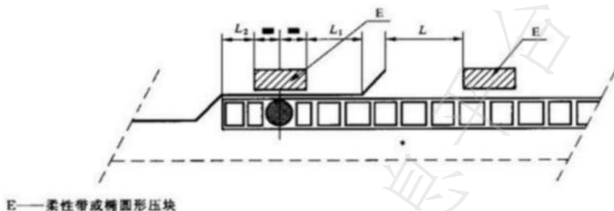
图A.3 再连接密封处压块的定位
